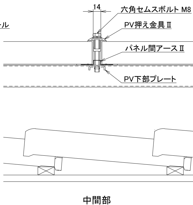
側面図
