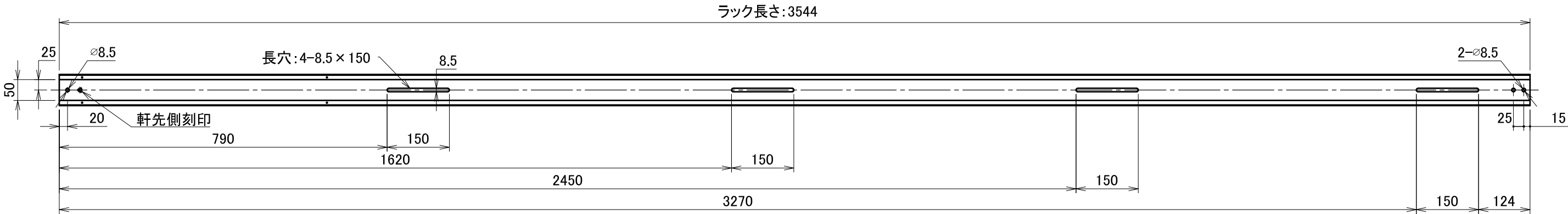
〈 ラック天面 穴詳細図 S:1/10 〉
