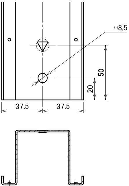
〈 軒先側刻印位置 S:1/2 〉
