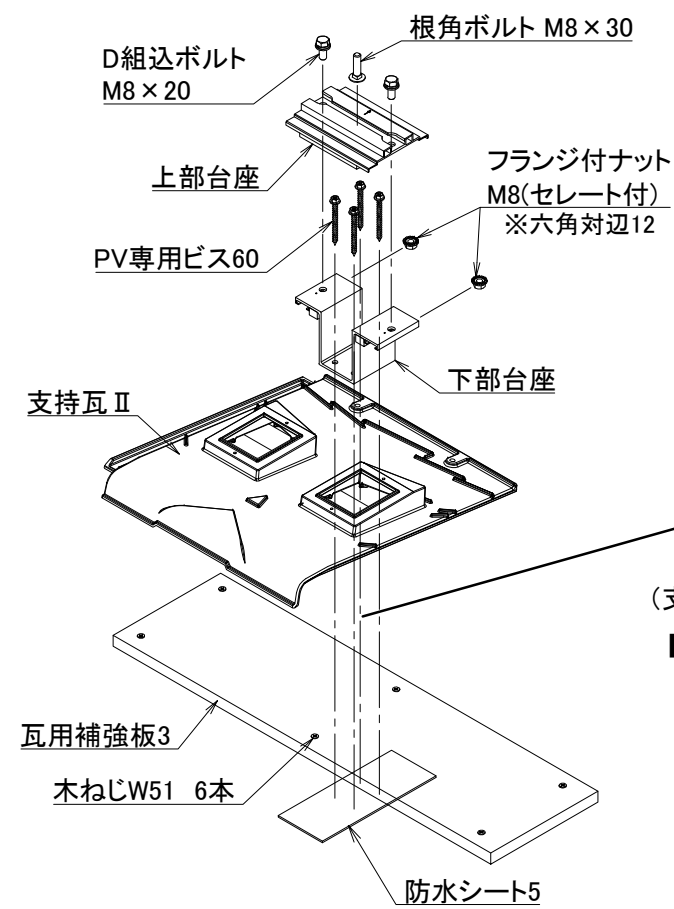
＜ 支持瓦Ⅱの取付 ＞ ■多雪セットの場合
