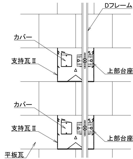
【1段飛ばし設置】
