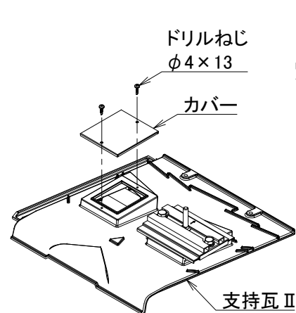
＜カバーの取付＞
