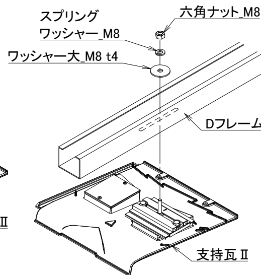
＜ Dフレームの取付 ＞
