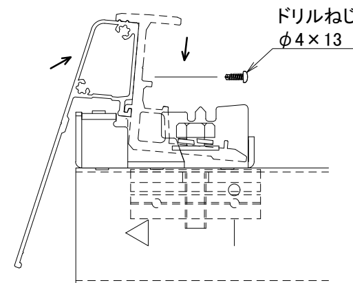
◎ ラック間アースⅡの取付
