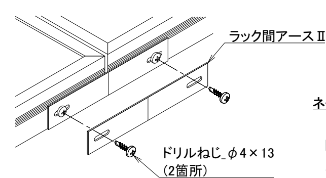
◎ ラック間アースⅡの取付
