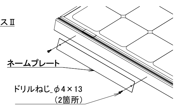
◎ ネームプレートの取付
