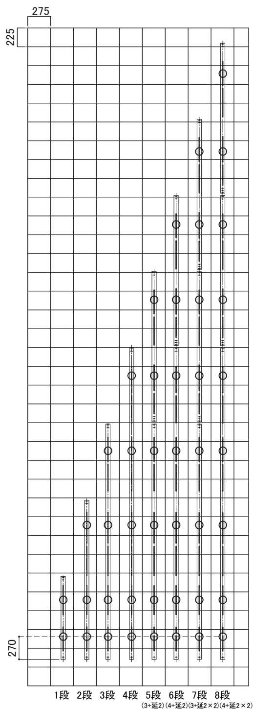
施工2・施工3 ※軒の出 270mm の場合 ※施工3／多雪区域：5段以上設置不可
