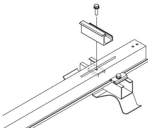
PV 端部押え金具の取付（棟側）
