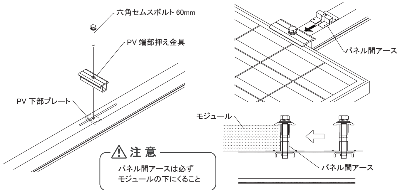
PV 押え金具の取付 (中間部)
