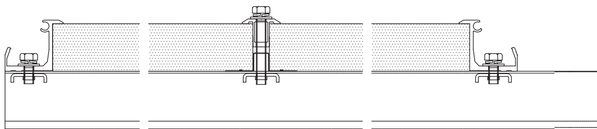
モジュール施工断面図
