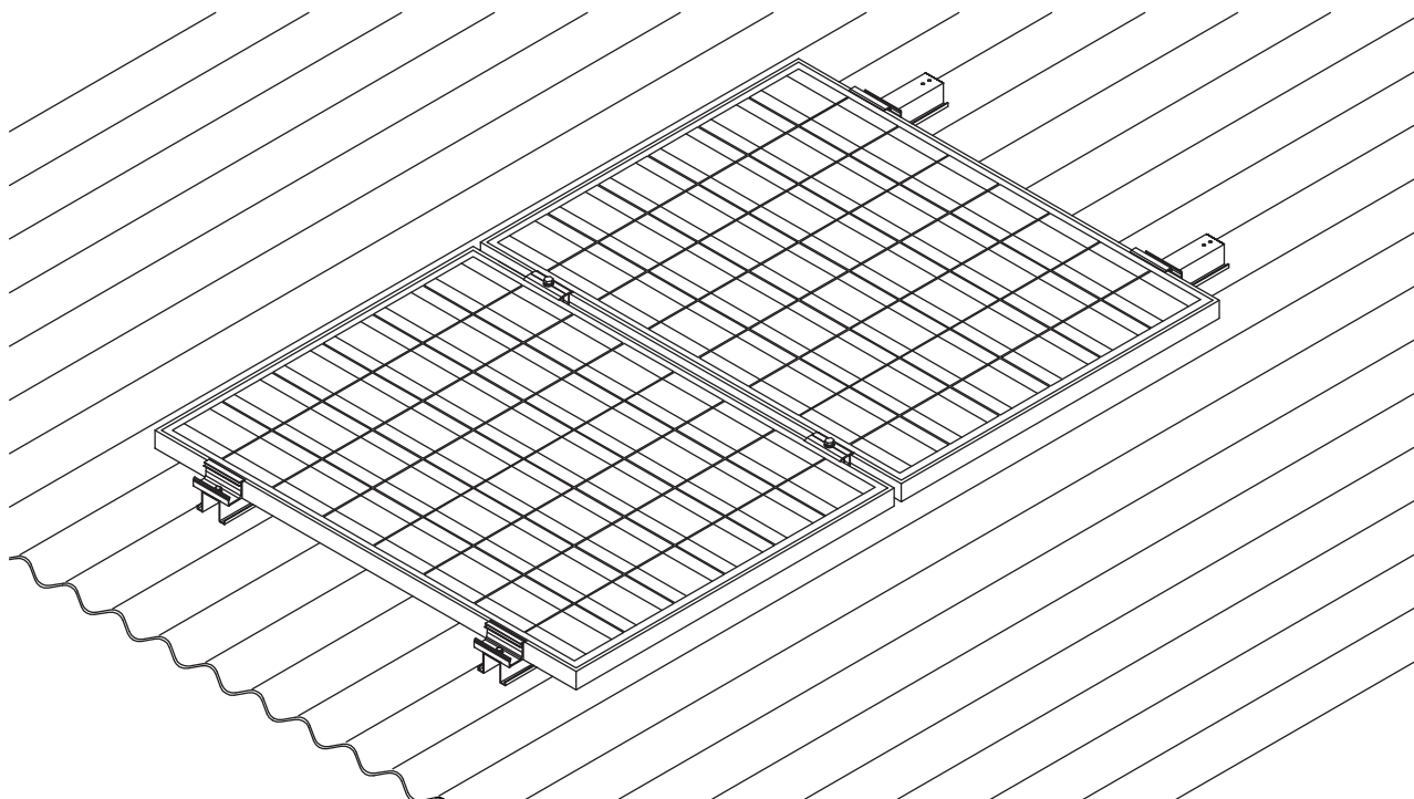
2 段目以降のモジュールの施工
