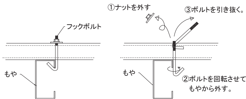
フックボルトの外し方
