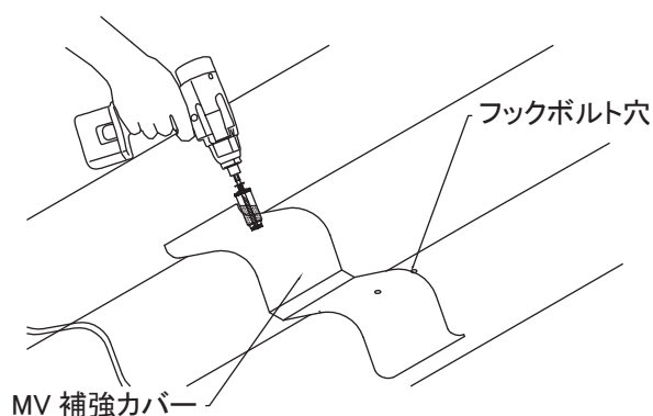
DHドリルで下穴穿孔
