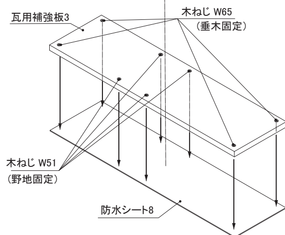
小幅板セットの場合
