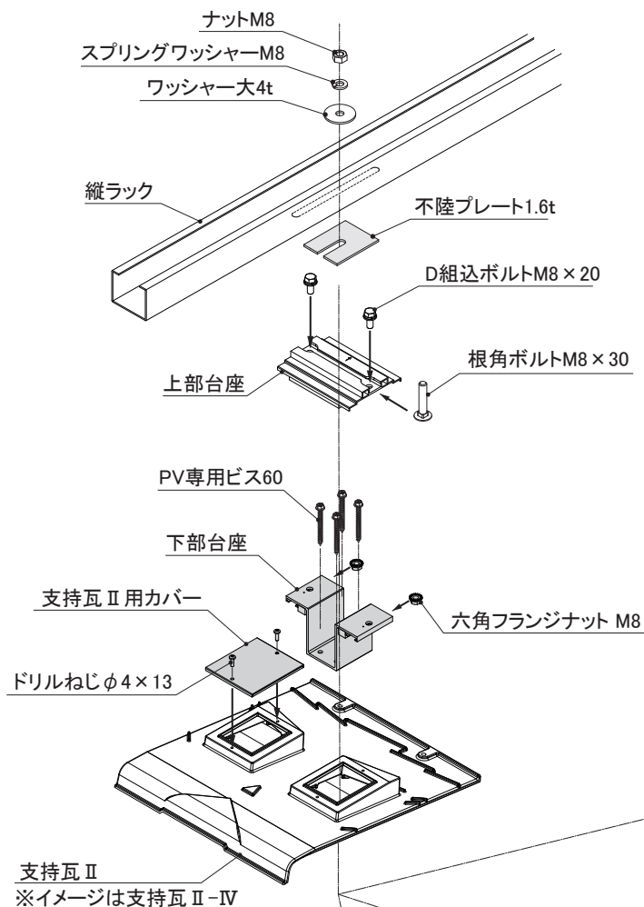
支持瓦Ⅱ仕様構成図(縦ラック取付まで)
