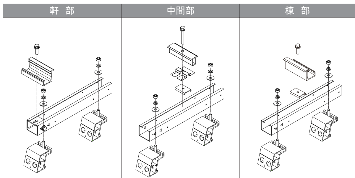
屋根材各部名称
