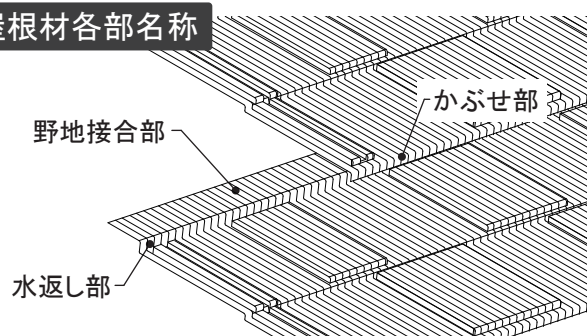
屋根斜視図
