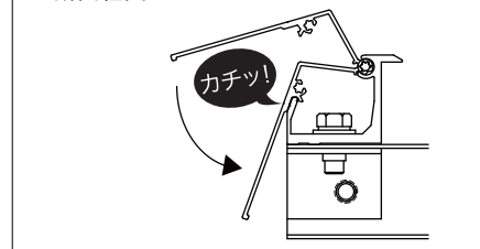
<断面組図>
