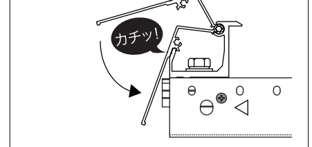
<断面組図>
