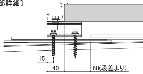
〔端部押え部詳細〕
