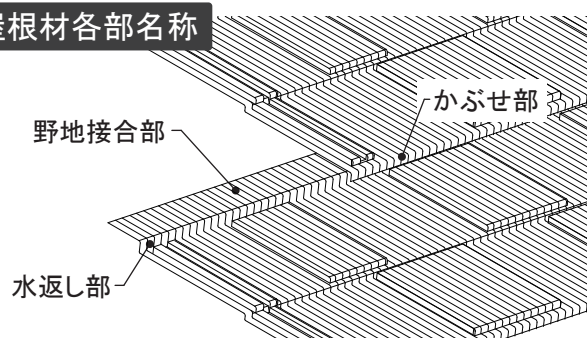
屋根斜視図
