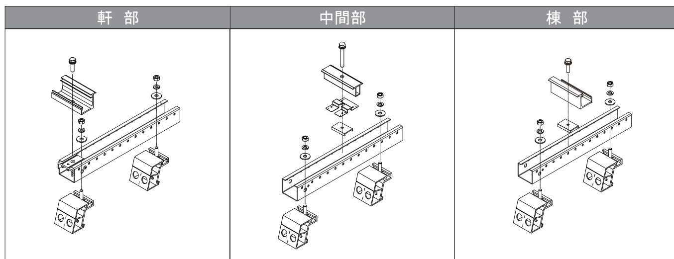
組立てイメージ
