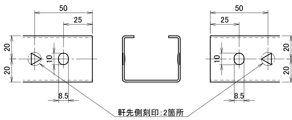
〈 D部 軒先側刻印位置 S:1/2 〉
