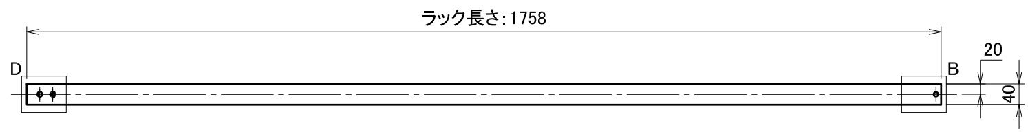
〈 ラック側面 ジョイント用穴詳細図 S:1/10 〉
