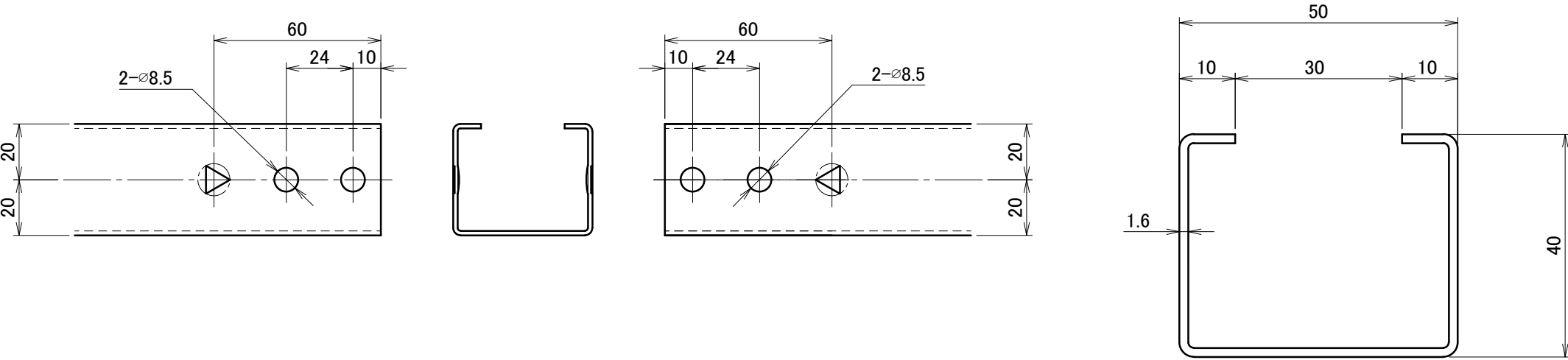
〈 D部 軒先側刻印位置 S:1/2 〉
