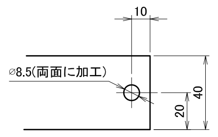
〈 B部詳細図 S:1/2 〉
