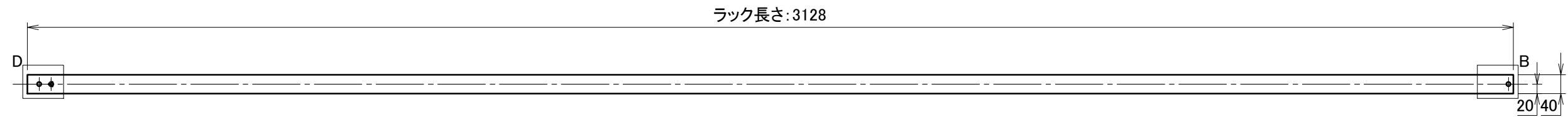
〈 ラック側面 ジョイント用穴詳細図 S:1/10 〉
