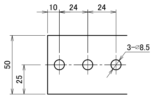
〈 C部詳細図 S:1/2 〉
