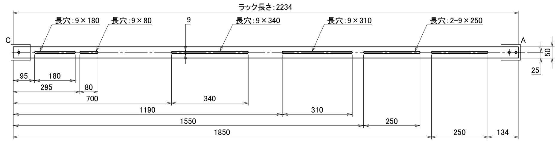
〈 ラック底面 長穴詳細図 S:1/10 〉
