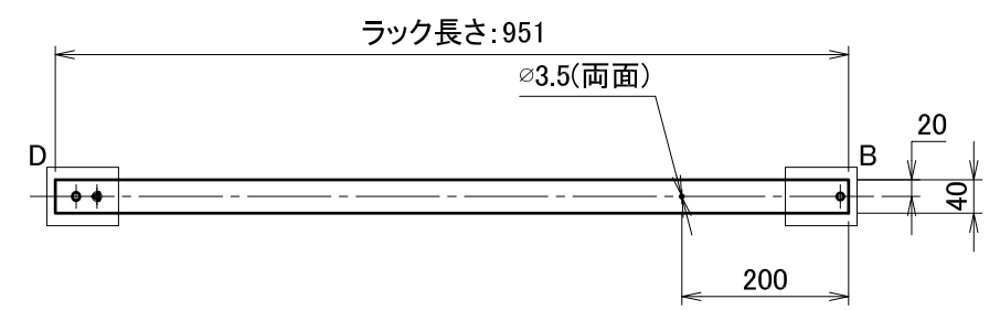
〈 ラック側面 ジョイント用穴詳細図 S:1/10 〉
