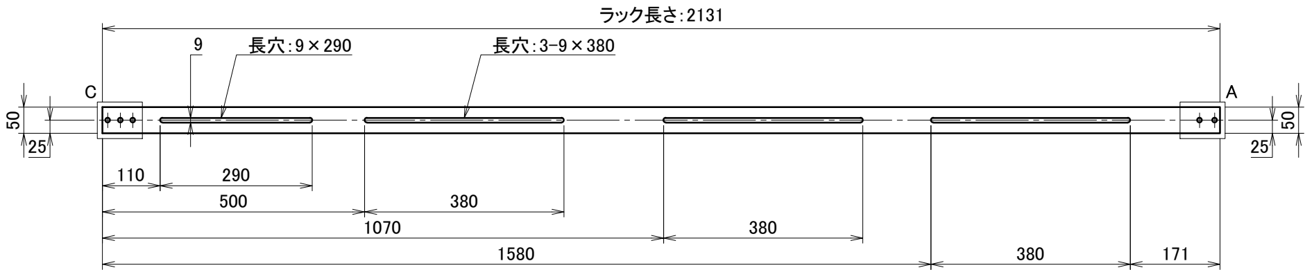
〈 ラック底面 長穴詳細図 S:1/10 〉
