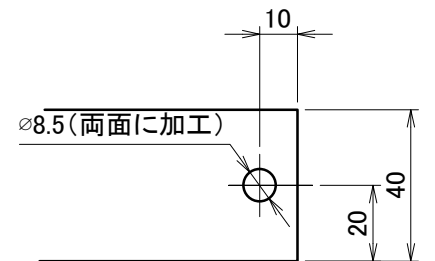
〈 B部詳細図 S:1/2 〉
