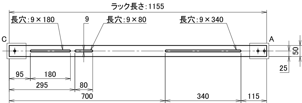
〈 ラック底面 長穴詳細図 S:1/10 〉
