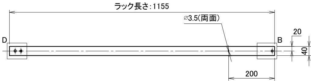
〈 ラック側面 ジョイント用穴詳細図 S:1/10 〉
