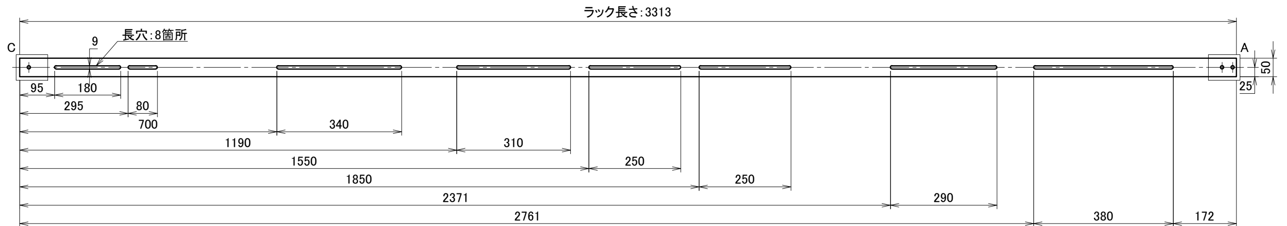
〈 ラック底面 長穴詳細図 S:1/10 〉
