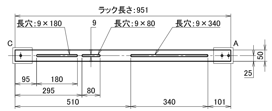
〈 ラック底面 長穴詳細図 S:1/10 〉
