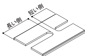
不陸用プレートⅡ（厚み 2.0mm）
