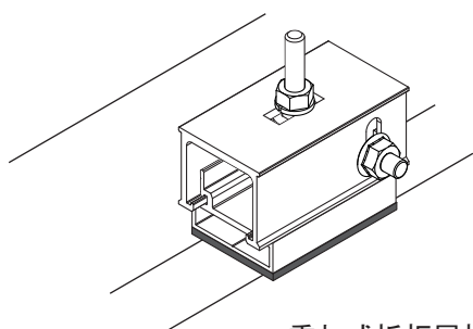
重ね式折板屋根用金具 DKS1-4
