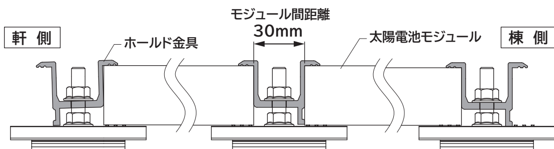
〔納まり図〕
