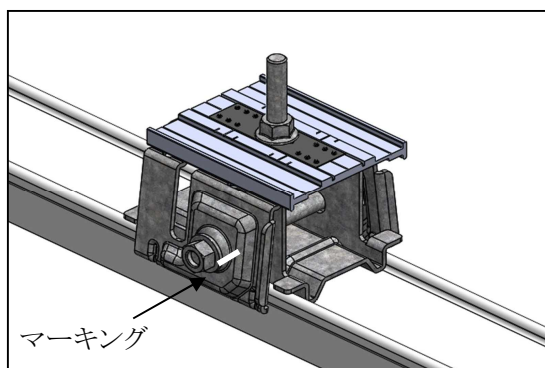
瓦棒丸ハゼ、林式瓦棒45・55
