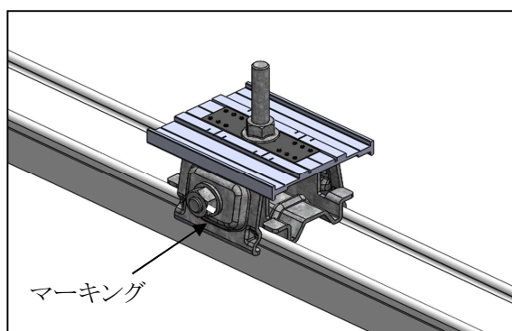
三晃式瓦棒
