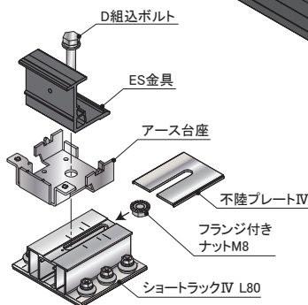
〔中間・棟部〕
