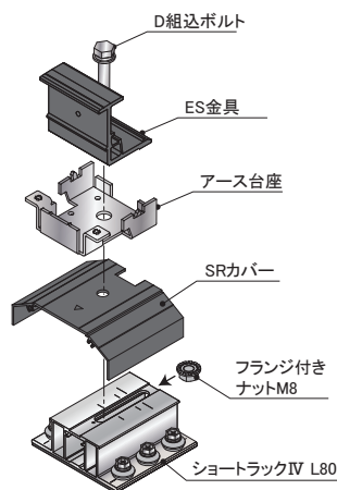
〔軒部〕
