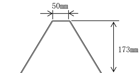
折板S60
